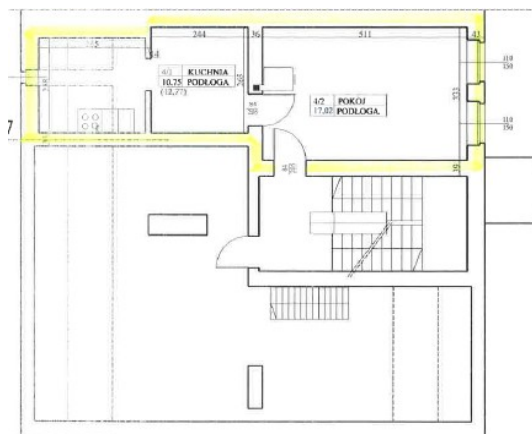
Rzut poddasza
